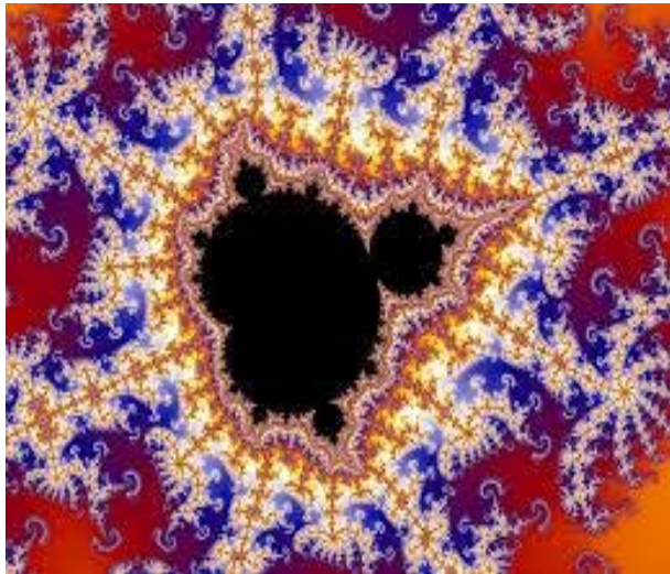
Fraktal
